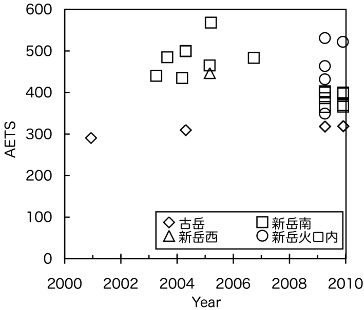
図 1 見かけの平衡温度 (AETS: \text{SO}_2+3\text{H}_2=\text{H}_2\text{S}+2\text{H}_2\text{O} )
