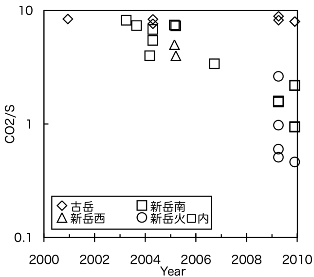
図 3 火山ガス中 CO 2 /S 比
