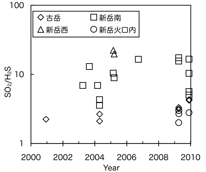
図 2 火山ガス中 SO 2 /H 2 S 比
