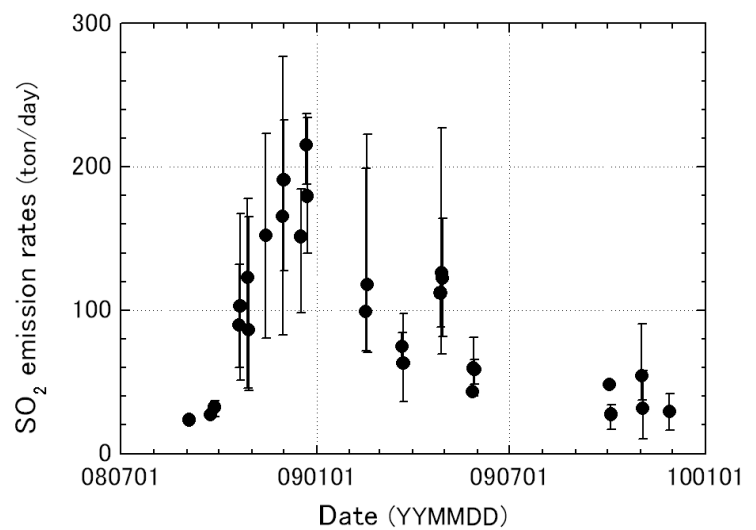
図 4 SO 2 放出量
