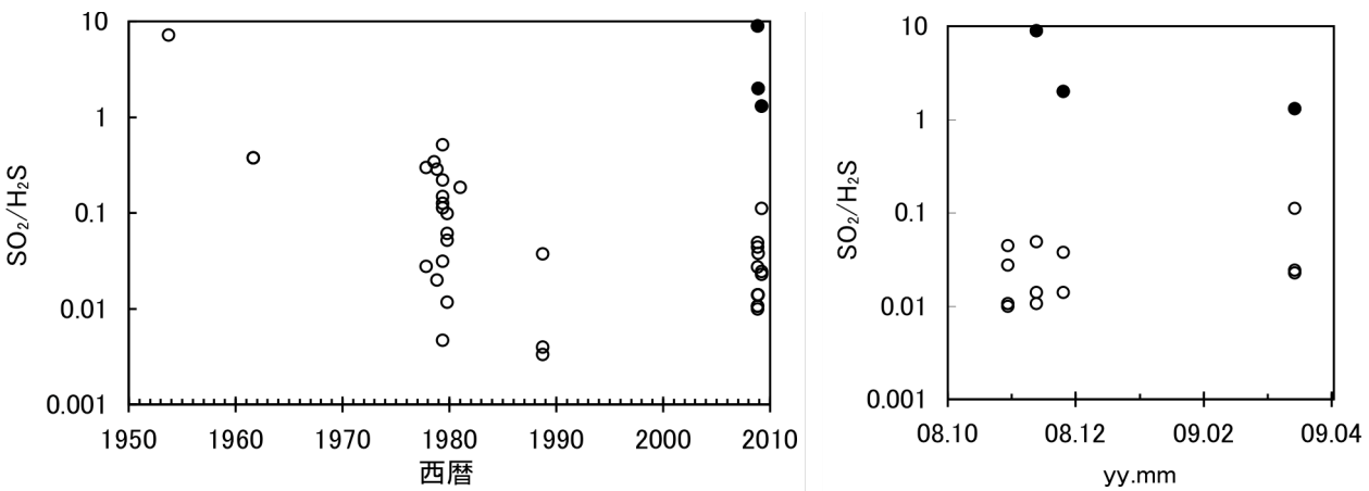
図 3 火山ガス中 SO_2/H_2S 比 (黒丸は新噴気)
