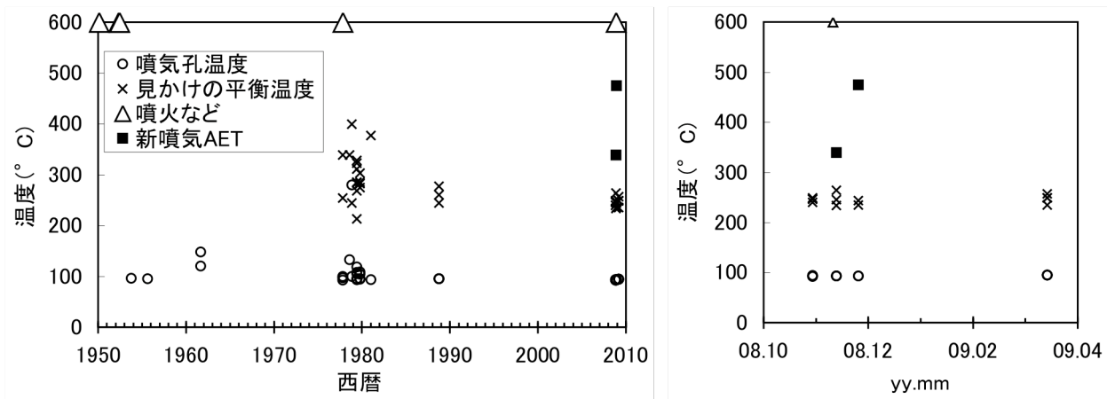
図 1 噴気温度と見かけの平衡温度 (AET: SO_2+3H_2=H_2S+2H_2O )
