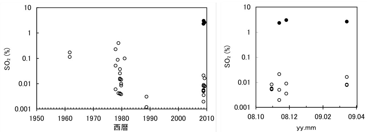
図 2 火山ガス中 SO_2 濃度 (黒丸は新噴気)
