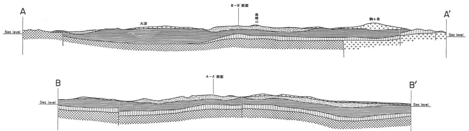
第13-1 仙岩地域地質編集図
