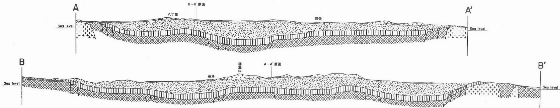
第24-1図 豊肥地域地質編集図
