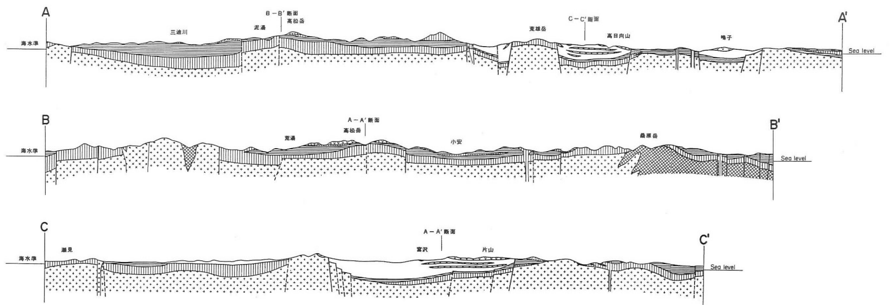
第14-1図 栗駒地域地質編集図
