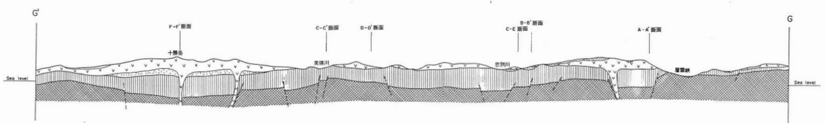
第4-1図 大雪山地域地質編集図
