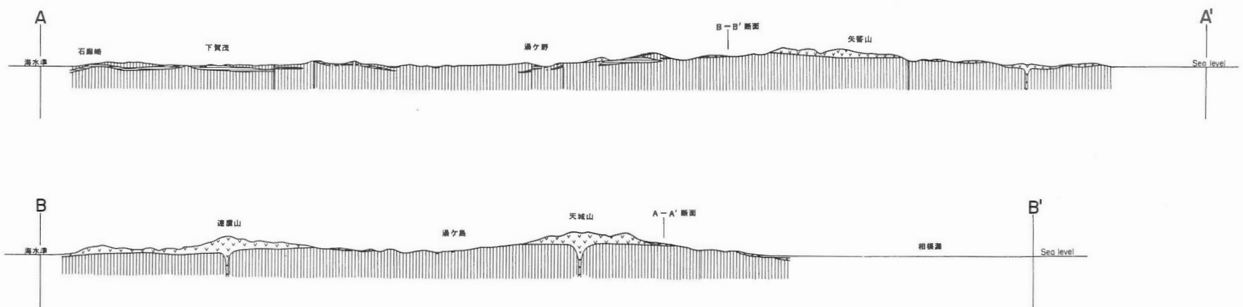
第23-1図 伊豆地域地質編集図
