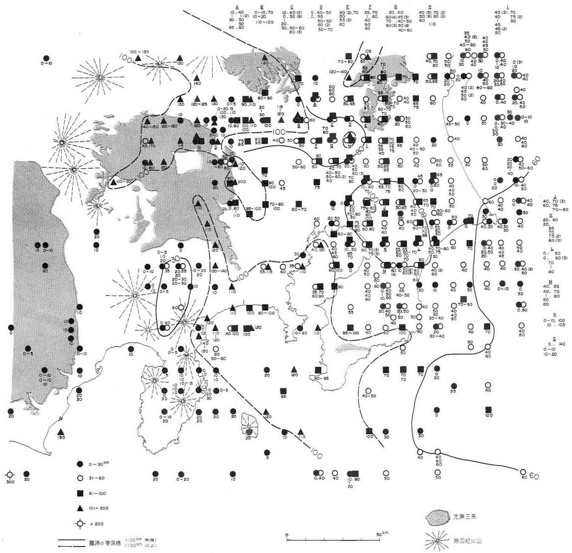
第16図 関東地方の震源分布図
