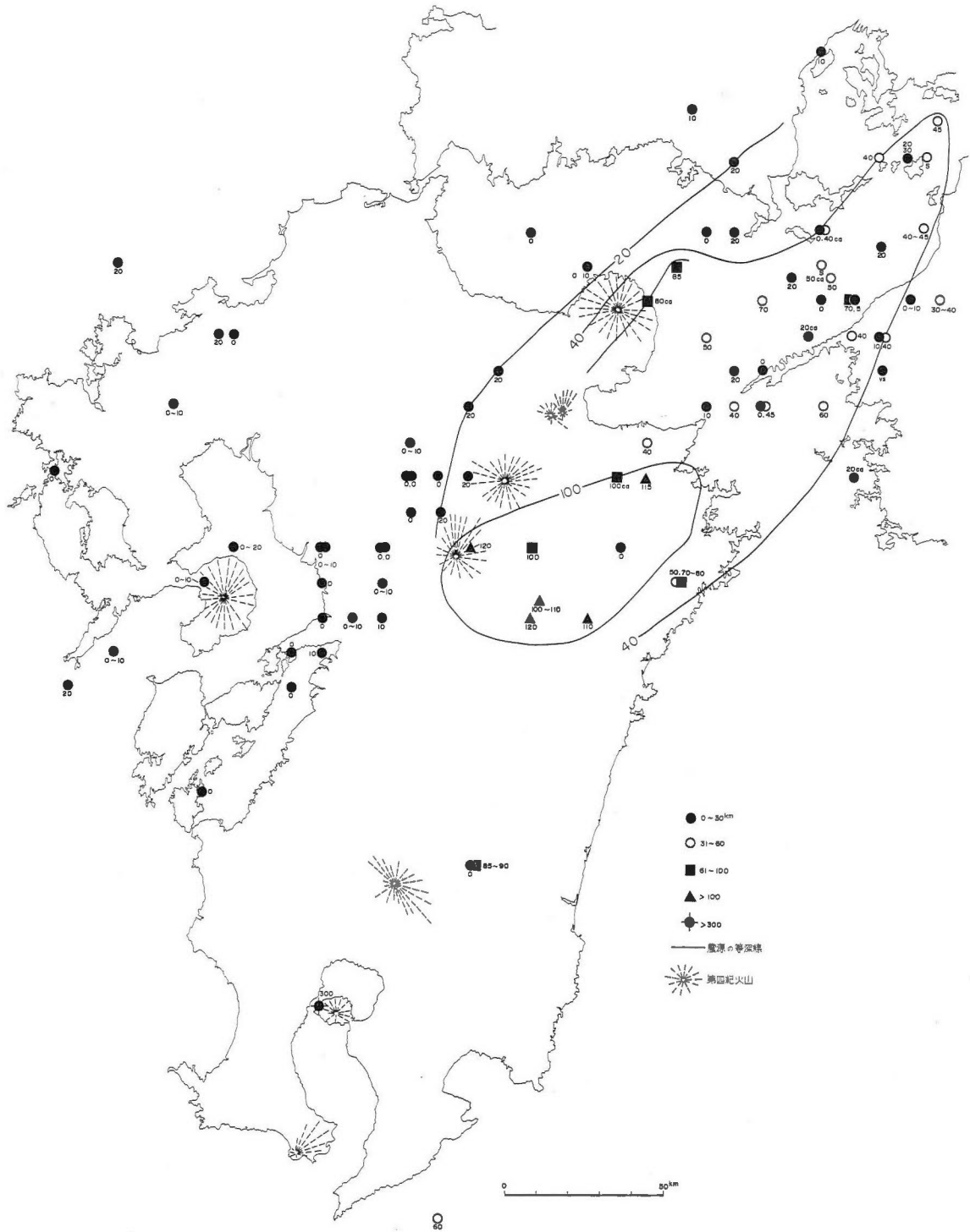
第23図 九州地方の震源分布図
