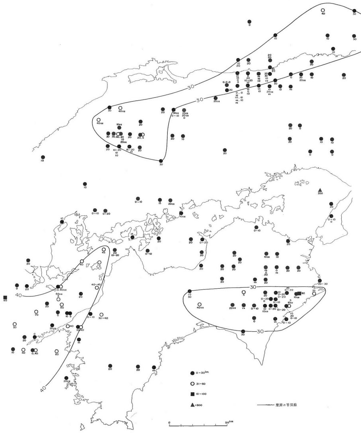
第22図 中国・四国地方の震源分布図
