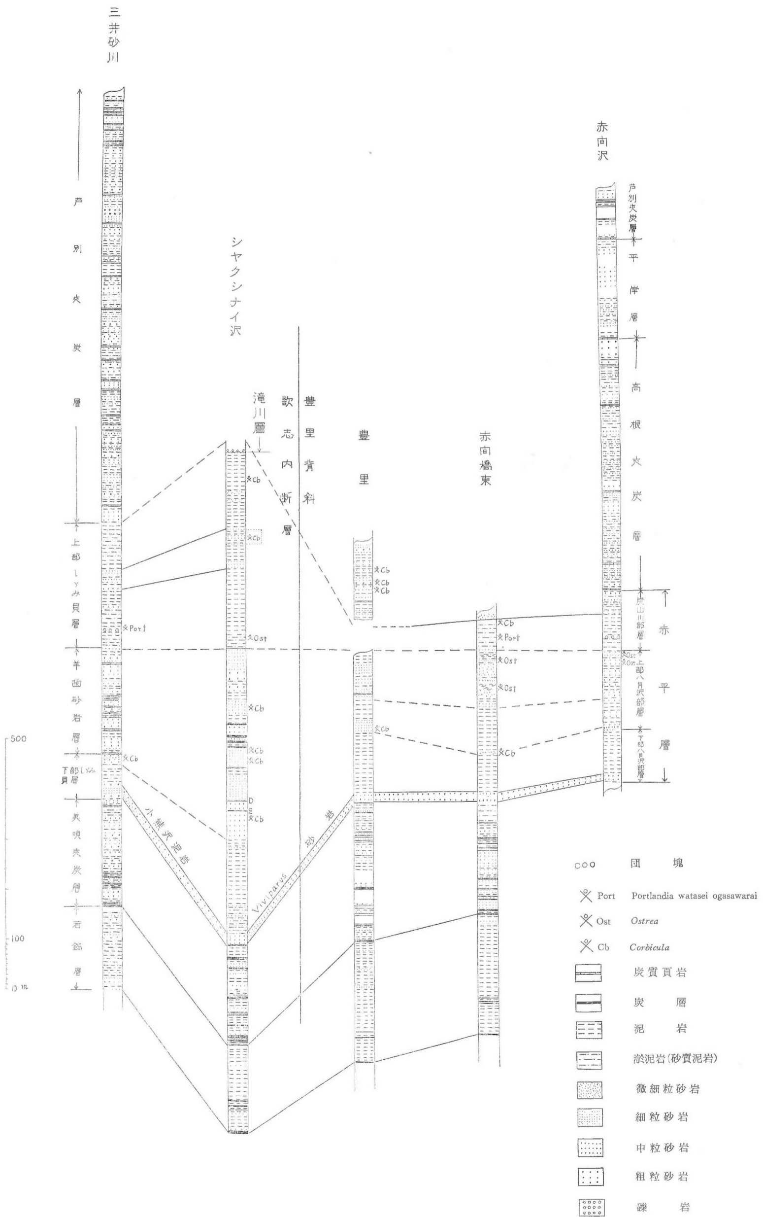
第3図 豊里背斜東西両翼の対比案 A (東翼の赤平層と西翼の上部しづみ貝層の各海成部位を同層準とみなした場合)
