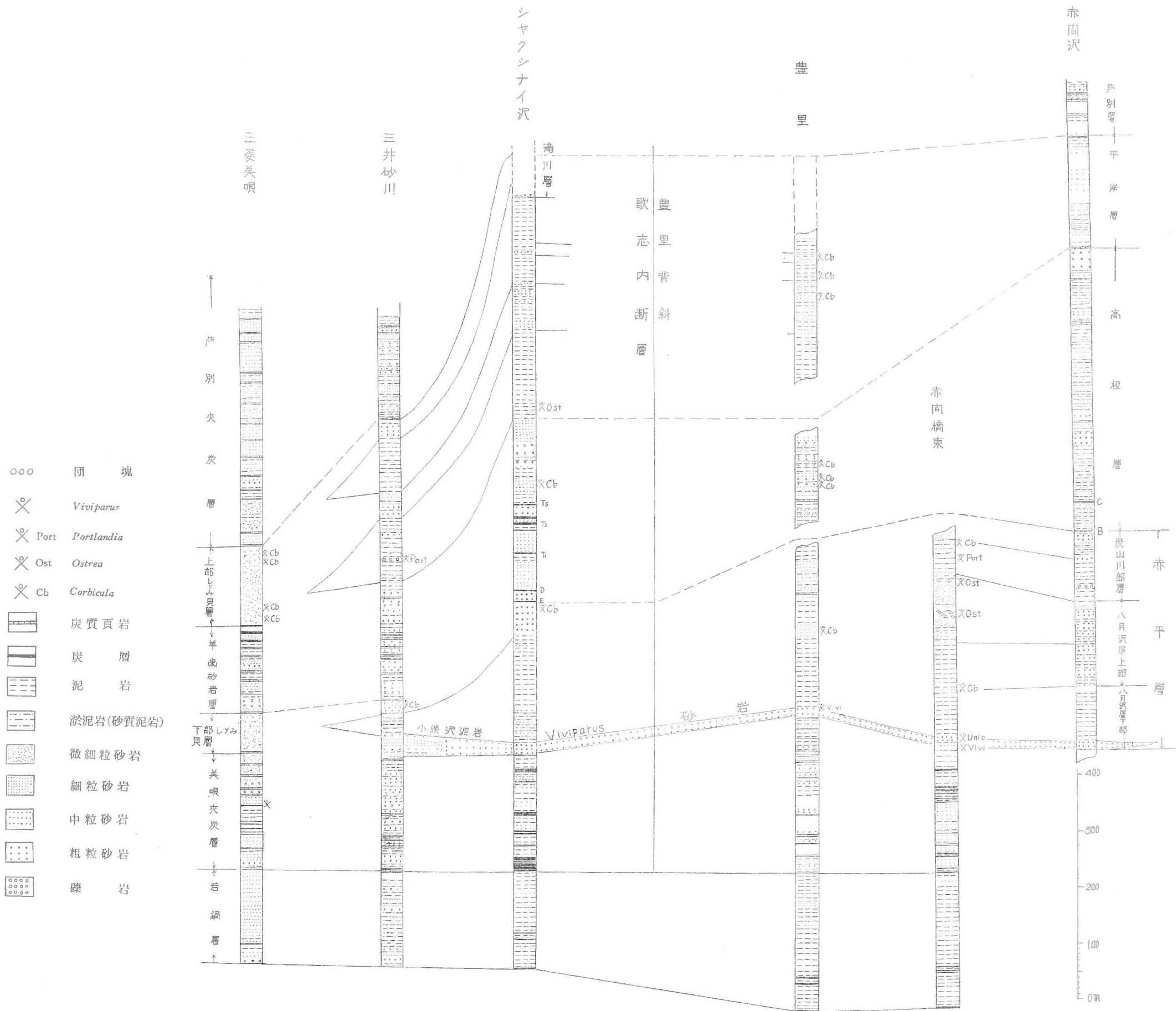
第4図 豊里背斜東西両翼の対比案 B (東翼の赤平層と西翼の上部しづみ貝層の各海成部位を同層準とみなさない場合)
