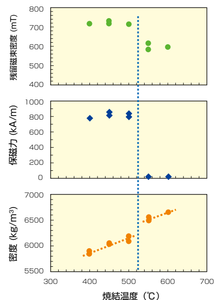
図1 Sm-Fe-N粉末の焼結温度と残留磁束密度 (Br)、保磁力 (Hcj) および焼結密度の関係 点線の温度付近でSm-Fe-Nの分解が occurring している。
