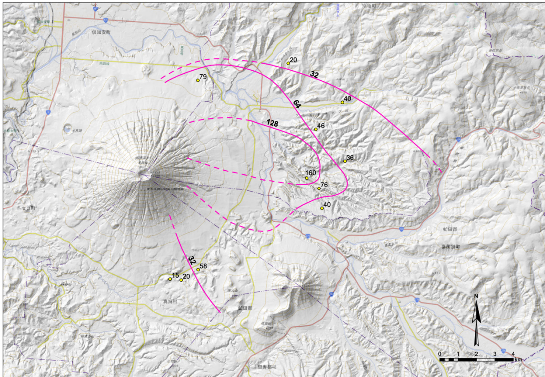
図 8. 羊蹄 Y26 降下テフラの等層厚線(Uesawa et al. , 2016)を GIS 化した図。実線は实在部分、破線は推定部分、黄色の点は各地点での層厚を示す。厚さの単位は cm。背景地図は国土地理院発行の地理院地図(標準、陰影起伏図)を使用した。
