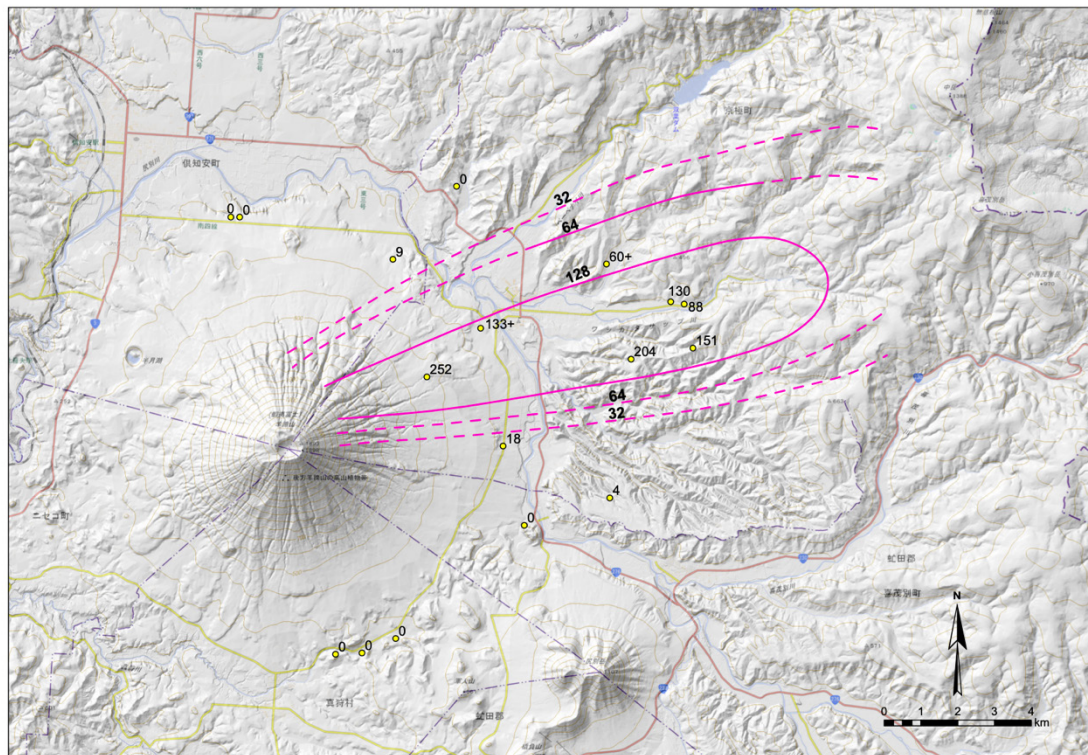
図 5. 羊蹄 Y11 降下テフラの等層厚線(Uesawa et al. , 2016)を GIS 化した図。実線は实在部分、破線は推定部分、黄色の点は各地点での層厚を示す。厚さの単位は cm。背景地図は国土地理院発行の地理院地図(標準、陰影起伏図)を使用した。
