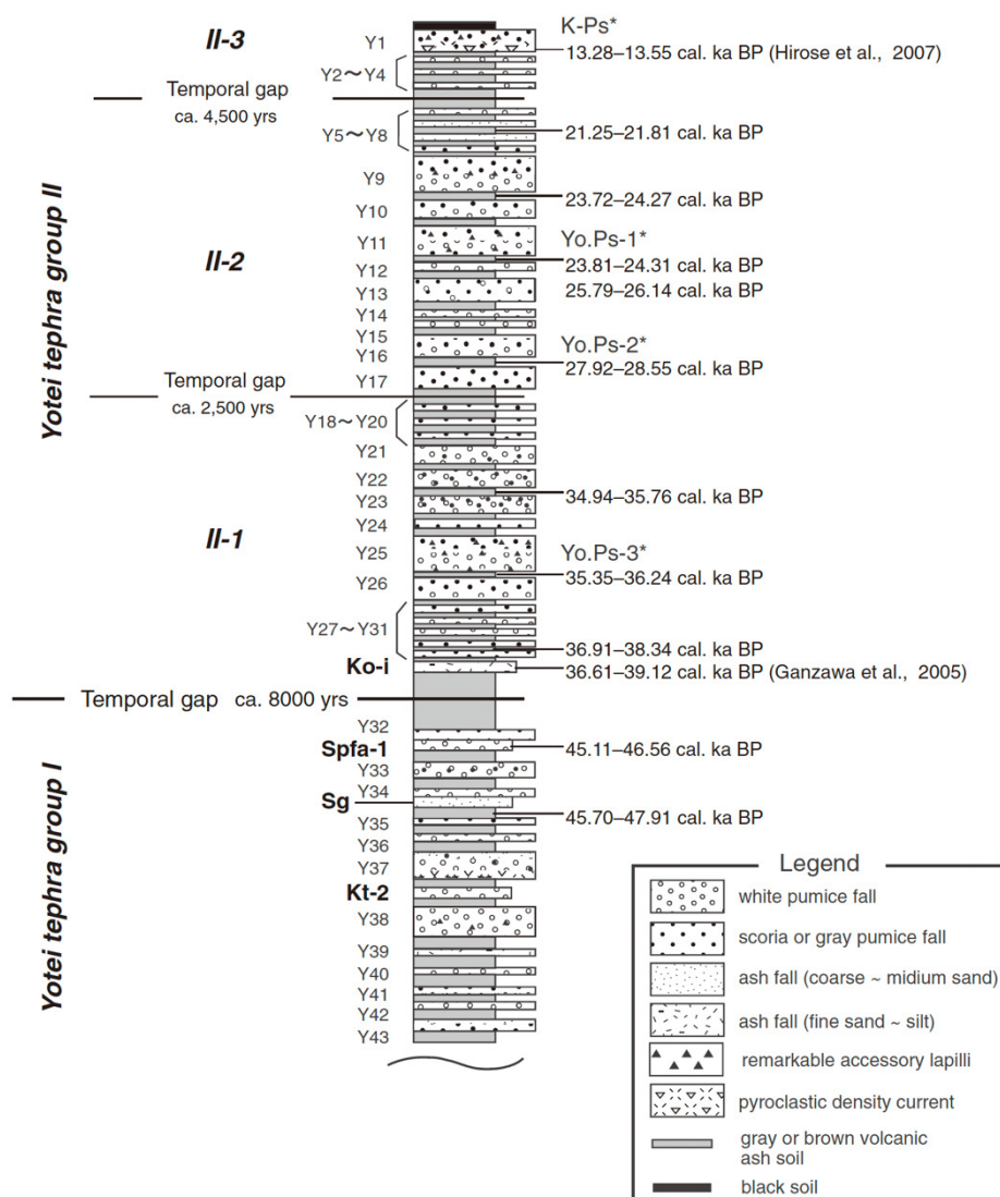
図 1. 羊蹄火山山麓付近の降下テフラ群の模式柱状図 (Uesawa et al. , 2016). K-Ps, Yo.Ps-1, Yo.Ps-2, Yo.Ps-3 は柏原ほか(1976)による名称. Ko-i: 北海道駒ヶ岳 Ko-i 降下テフラ. Spfa-1: 支笏第 1 降下テフラ. Sg: しおがま状降下テフラ. Kt-2: クッタラ第 2 降下テフラ. Fig. 1. Tephrostratigraphic column for units around the base of Yotei Volcano (Uesawa et al. , 2016). Ko-i: Hokkaido-Komagatake Ko-i tephra fall deposit. Spfa-1: Shikotsu 1 tephra fall deposit. Sg: Shiogamajyo tephra fall deposit. Kt-2: Kuttara 2 tephra fall deposit.
