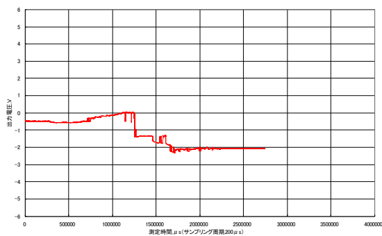
図 6-8 測定結果 4 (標準)
