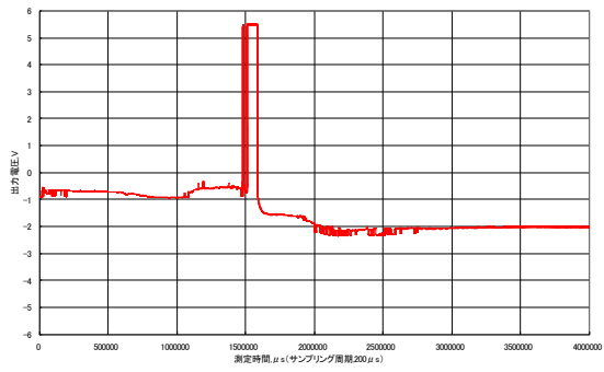
図 6-9 測定結果 5 (標準)
