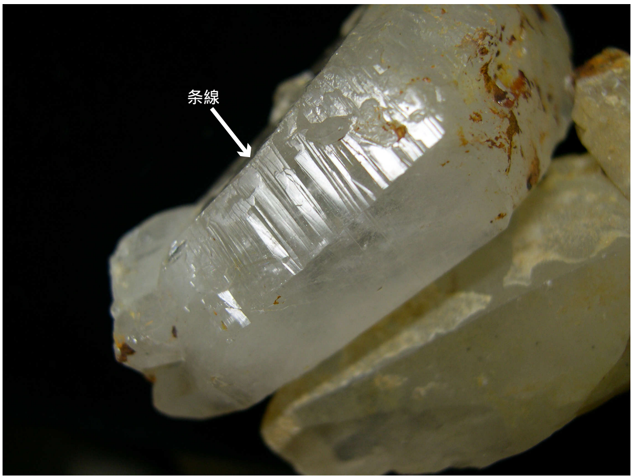
水晶 茨城県桂村錫高野 六角柱状の結晶．結晶の伸びの方向に対して垂直な方向に条線が見られる．結晶の長さ約4cm
