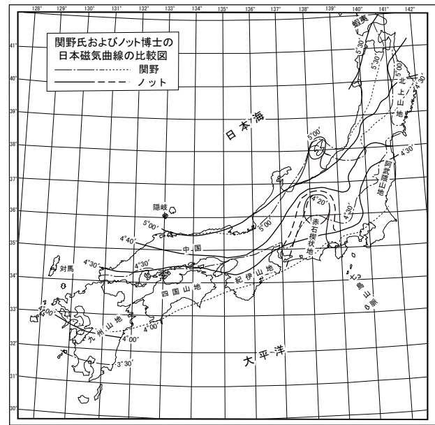
第4図 関野氏およびノット博士の日本磁気曲線の比較図. 関野らの観測による等偏角線図(Naumann, 1887a)とノットらの等偏角線図(Knott and Tanakadake, 1888)を比較するために, ナウマンが作成したもの. 原図を約65%に縮小. ノットらの等偏角線図のうち, 北陸海岸に沿って延びる5°Wの曲線と佐渡を取り囲む5°Wの閉曲線とを繋ぐ2本の曲線およびその南方の4°20'W [4°30'Wの誤り]の閉曲線東縁から南方に延びる曲線は, ナウマンが書き加えた部分である.
