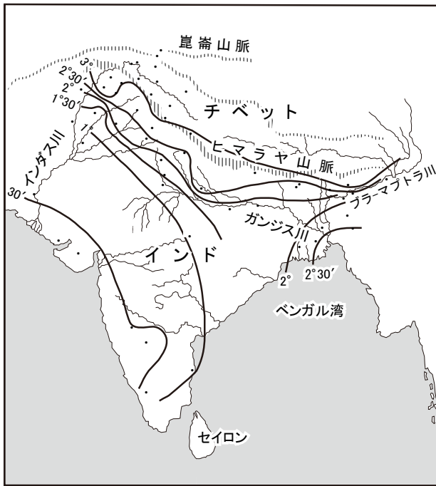
第2図 インド-ヒマラヤ地方の等偏角線図. Rijckevorsal (1879)の観測データに基づいてナウマンが作成したものを和訳した。原図を約70%に縮小。偏角値は西偏を、黒点は観測点(観測値は省略)を、ケバは主要な山稜を示す。ブラマプトラ川の地名を追記した。
