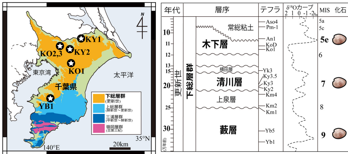
第1図 千葉県の地質図(左)と下総層群の層序(右)。左図：オレンジ色の部分が下総層群の分布域です。星マークは本研究に用いた化石標本の産出地点を示しています。右図：貝のマークは、木下層、清川層、藪層からピノスガイが見つかることを意味します。※原論文の図を引用・改変したものを使用しています。
