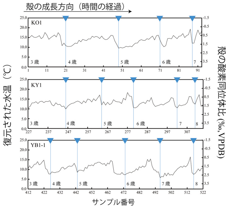
第3図 木下層から産出したビノスガイの化石 (KO1)，清川層から産出したビノスガイの化石 (KY1)，藪層から産出したビノスガイの化石 (YB1) が若いころに経験した水温の季節変動の復元結果。青い三角形と青い線は1年間の区切りである年輪の位置を意味し、線と線の間が1年間です。水温復元の計算に必要な当時の海水の塩分は、現在の岩手県沿岸の外洋の塩分と同程度と仮定しています。分析による復元水温の誤差は±1℃未満です。※原論文の図を引用・改変したものを使用しています。
