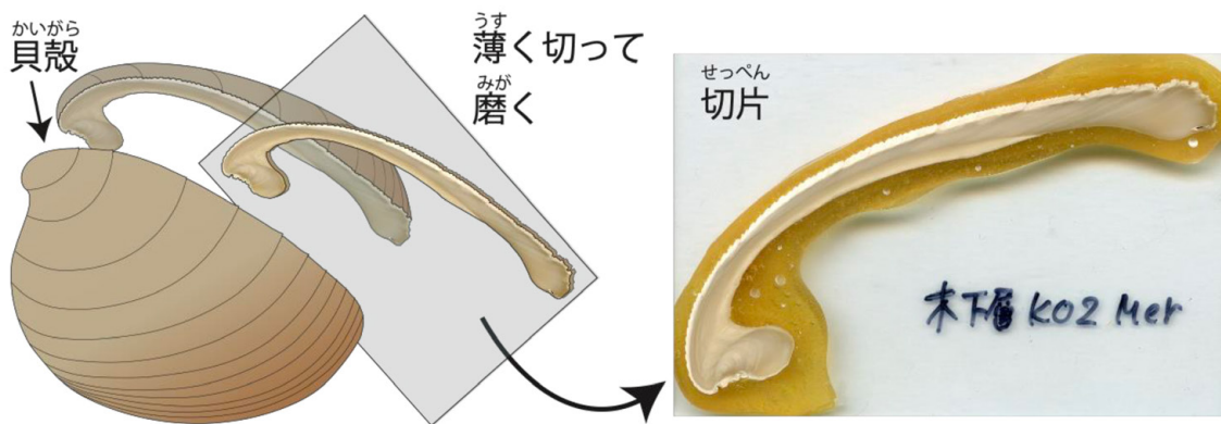
第2図 101歳の化石ピノスガイの貝殻をスライスして研磨した切片試料。
