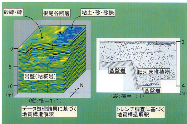
2. 3次元反射法探査結果に対する地質構造解釈。
