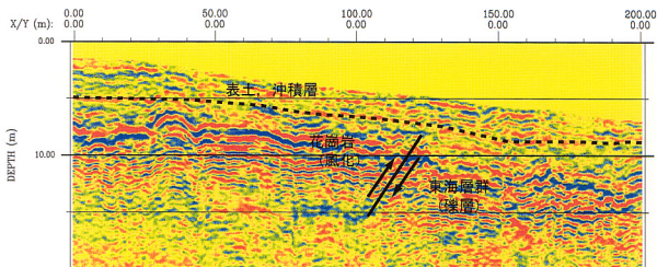
1. GPR反射法探査による記録断面から得た地質構造解釈。
