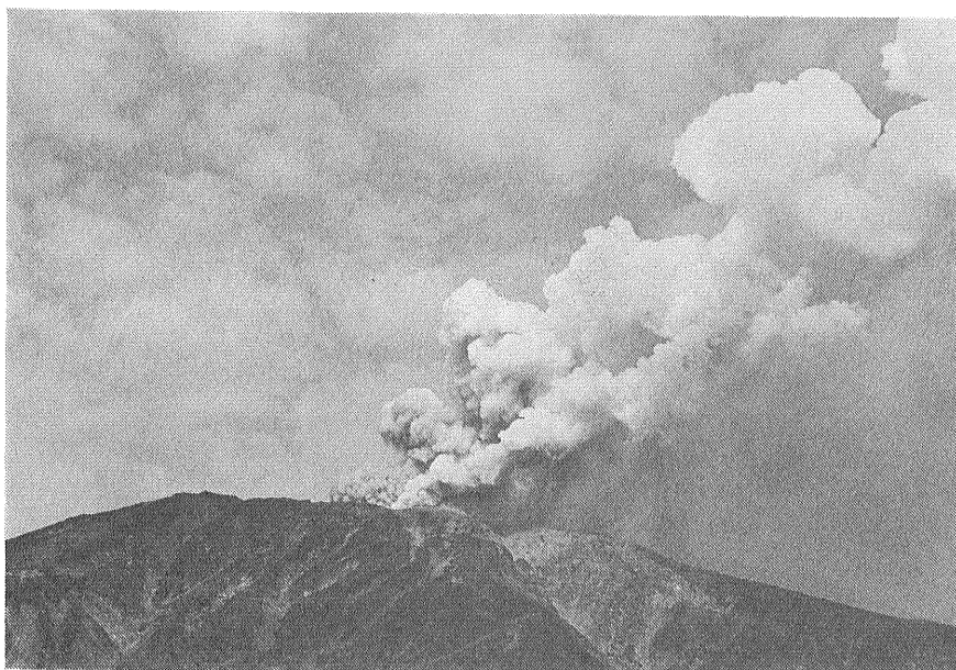
写真2 10月28日午前10時頃 御岳山7合目田の原高原からみた噴煙 噴煙の低位左半分は灰色を呈し主火口から噴出したもの 写真右側の白煙の下にカーテン状に降灰が認められる（春日井市 井上栄さん撮影）
