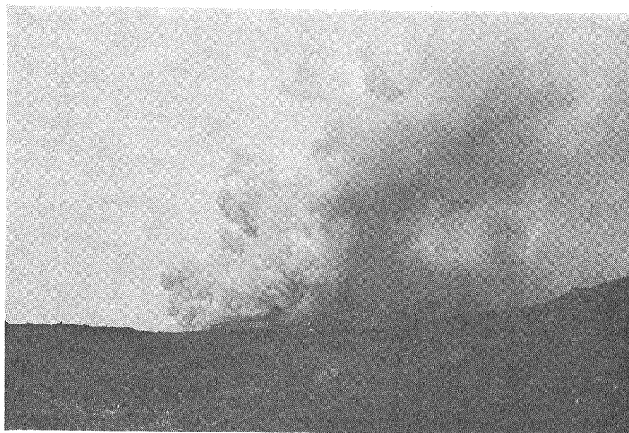
写真 1 10月28日午前 8 時 30 分頃 王滝山頂まで 600m の位置 から見た噴煙 (春日井市 井上栄さん撮影)
