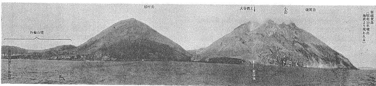
硫 黄 島 の 主 要 部 (島の南方海上から中央火口丘を望む)
