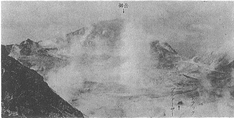
硫黄岳の火口 〔向う側は最高峯御岳(703m)〕 火口底内で ブルドーザーやトラックが硫黄を採掘し運搬している
