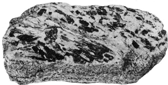
亜灰長石・エディン石・直閃石・パーガス石片麻岩 (Bytownite-Edenite-Anthophyllite-Pargasite Gneiss)
