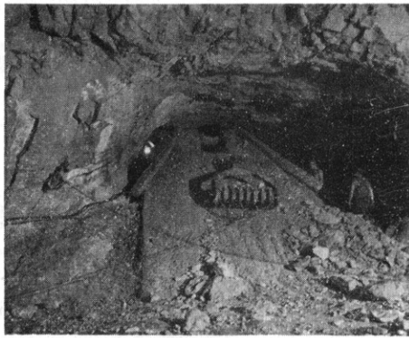
坑内のスクレーパー操作
