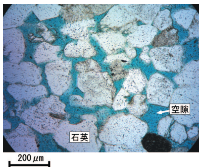
口絵1: 米国産の砂岩(ベリア砂岩)の薄片の偏光顕微鏡写真(オープンニコル)。空隙は, 青色の樹脂が圧入してあるので, この写真では青色として写っています。鉱物のほとんどは, 石英です。
