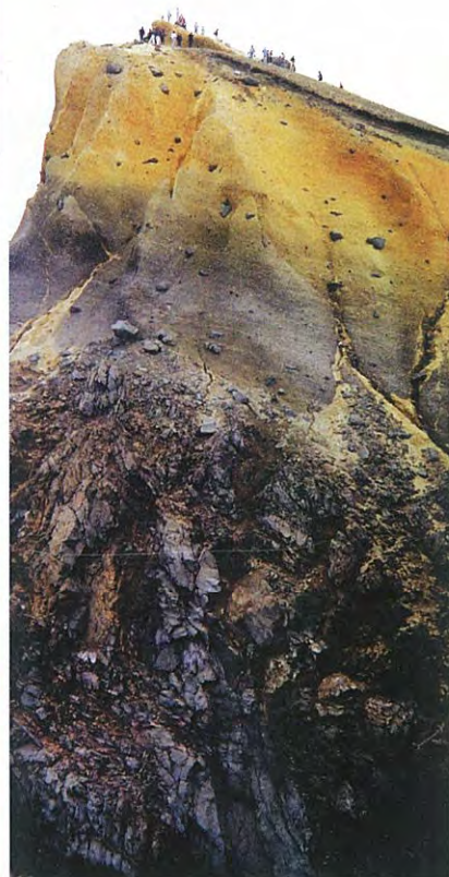
2. 長白山頂の断面。珪長質アルカリ岩類からなり、下部が溶岩、上部が凝灰岩。
