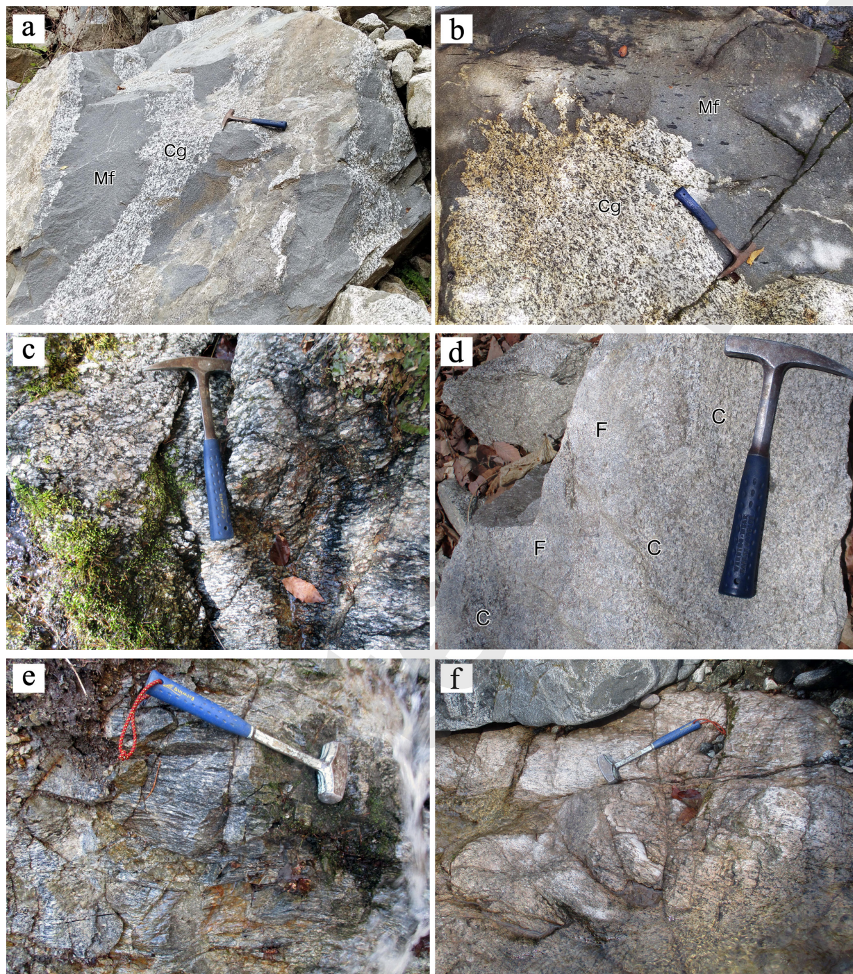
第3図 大河原地域に産する領家深成岩類の野外での産状。(a) 生田花崗岩粗粒相 (Cg)中の不規則な形態の苦鉄質岩類細粒相 (Mf)の包有物。Mfの文字のある包有物の境界は、写真(b)のような入道雲様を示す。(b) 生田花崗岩粗粒相 (Cg)と苦鉄質岩類細粒相 (Mf)の境界。境界部では、両岩相が相互に貫入し、入道雲様を示す。(c) 片麻状構造の発達する南向花崗岩粗粒相。(d) 南向花崗岩細粒相の産状。数cmの範囲で急激に粒度が変化し、粗粒部 (C)と細粒部 (F)とが不規則に分布する。(e) 縞状構造の発達する非持トータル岩。(f) 片麻状構造を示す生田花崗岩。
