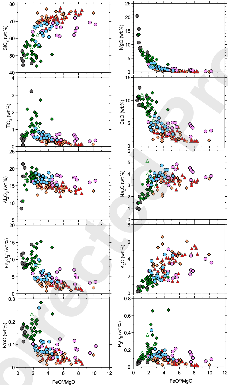
第7図 大河原地域に産する深成岩類の \text{FeO}^*/\text{MgO} に対する全岩主成分組成図。 \text{Fe}_2\text{O}_3^* は全鉄を \text{Fe}_2\text{O}_3 として、 \text{FeO}^* は \text{FeO} として示したもの。 凡例は第5図と同じ。
