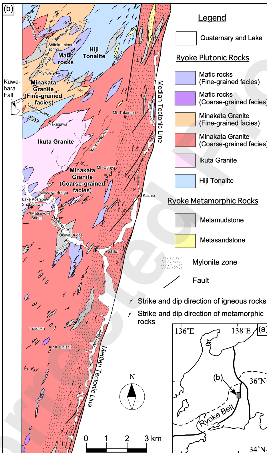
第1図 大河原地域の位置 (a)と領家深成変成コンプレックスの地質図 (b)。中央構造線の位置及びマイロナイト帯の分布とその中の構造ならびに第四系の分布は、中村ほか (2025) に基づく。地質単位・地名の日本語表記は付録に示した。
