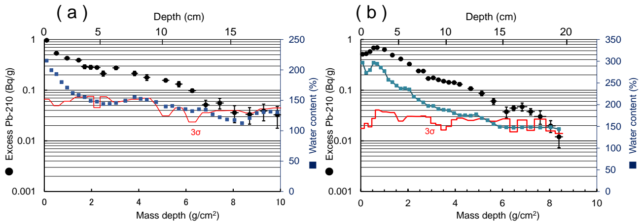
第 12 図 (a) コアA, (b) コアBにおける過剰 Pb-210と含水比の変化. 赤線は, 過剰 Pb-210の 3\sigma 検出限界を示す.
