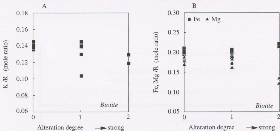
第8図 黒雲母の変質度に対する化学組成変化. RはSi+Al+Mg+Feのモル量を示す. A) 変質度に対するKとRのモル比. B) 変質度に対するFeまたはMgとRのモル比. 数字の0, 1, 2は各々新鮮, 弱, 中変質に対応する.
