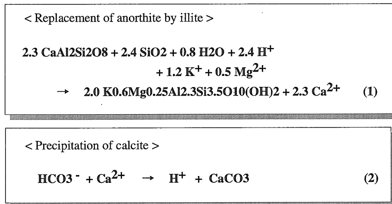
第10図 アノーサイトからイライトへの変質(1), および方解石の形成(2)の化学反応. (Hamasaki et al. , 1995). Fig. 10 Chemical reactions of alteration for anorthite to illite (1) and formation of calcite (2) (Hamasaki et al. , 1995).
