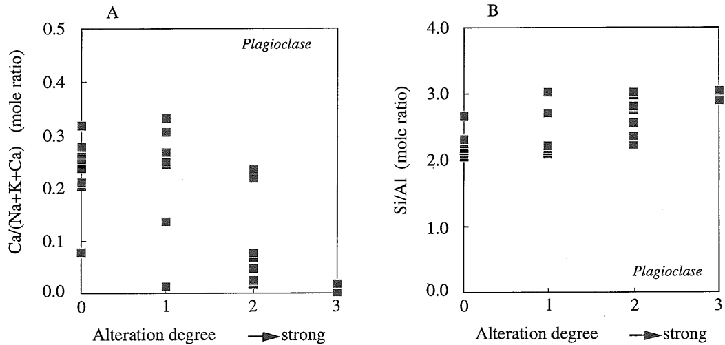
第9図 斜長石の変質度に対する化学組成変化. A) 変質度に対するCaとアルカリ元素のモル比. B) 変質度に対するSiとAlのモル比. Fig. 9 Chemical transition as an alteration degree of plagioclase. A) Calcium to alkali elements mole ratio as an alteration degree. B) Silica to aluminum mole ratio as an alteration degree.
