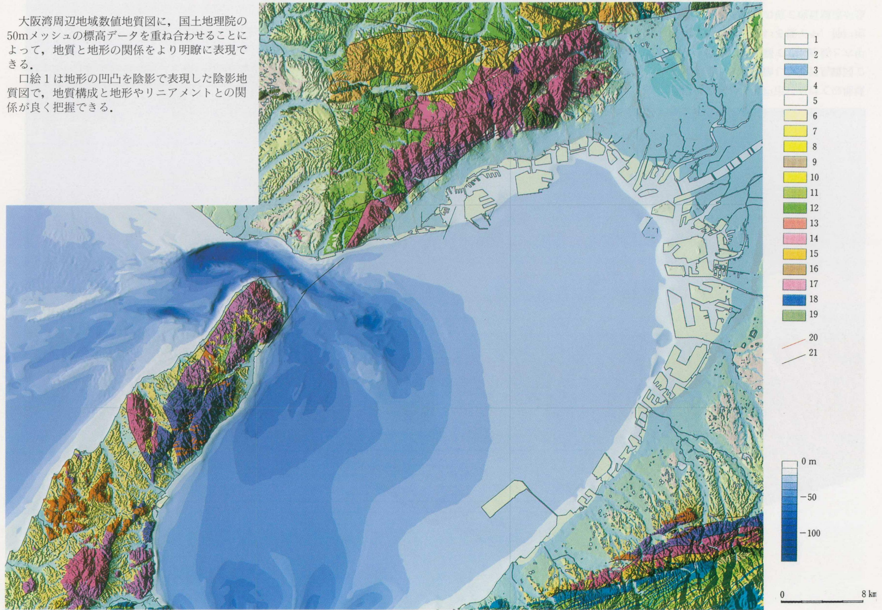
口絵1 大阪湾周辺地域の陰影地質図
