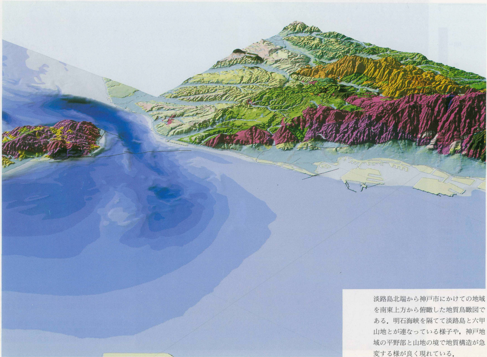
口絵2 大阪湾周辺地域の地質鳥瞰図
