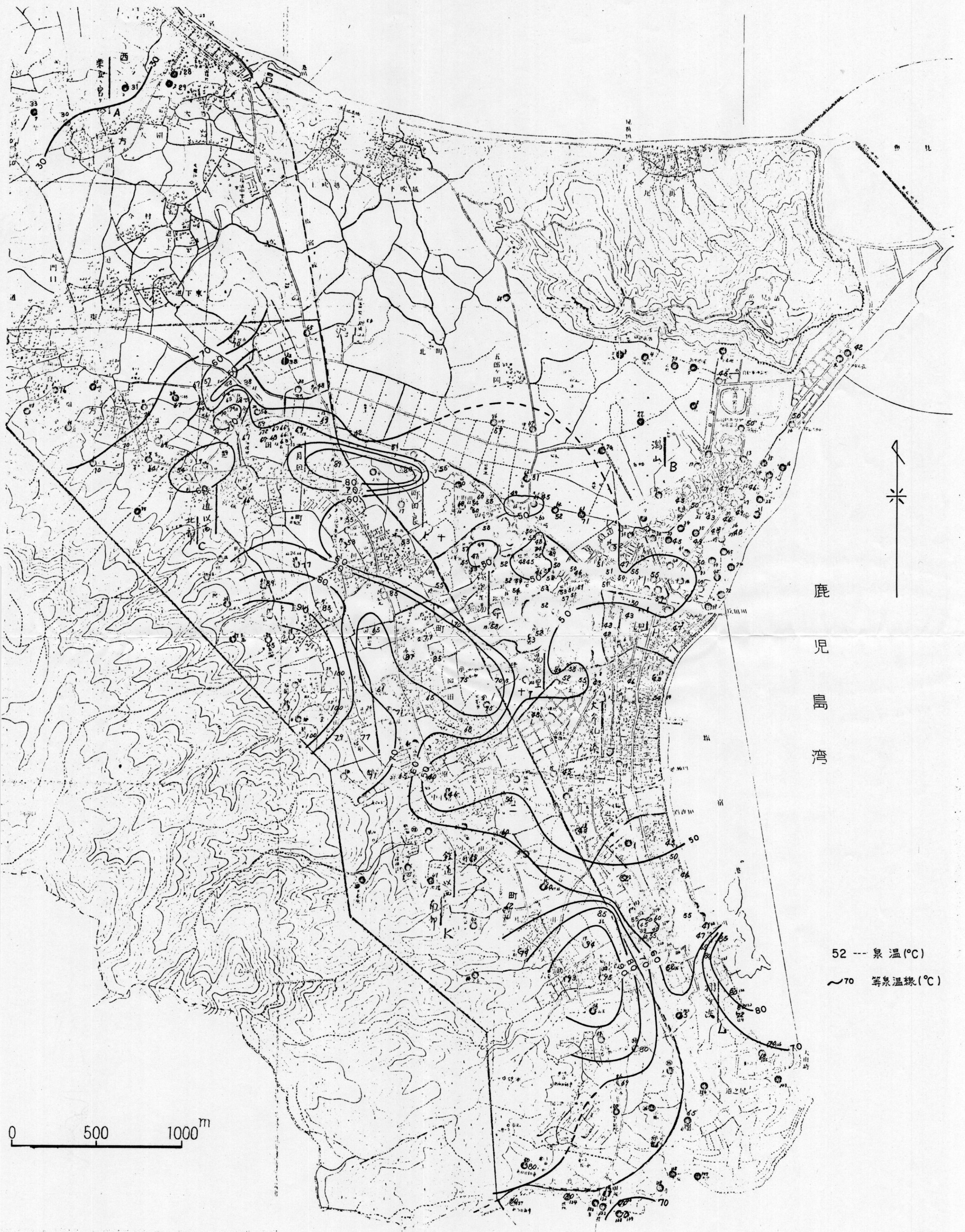
第20図 鹿兒島県指宿地域放熱量調査泉温分布図
