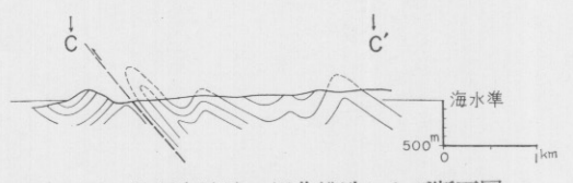
第1図 佐須奈地域の褶曲構造および断面図
