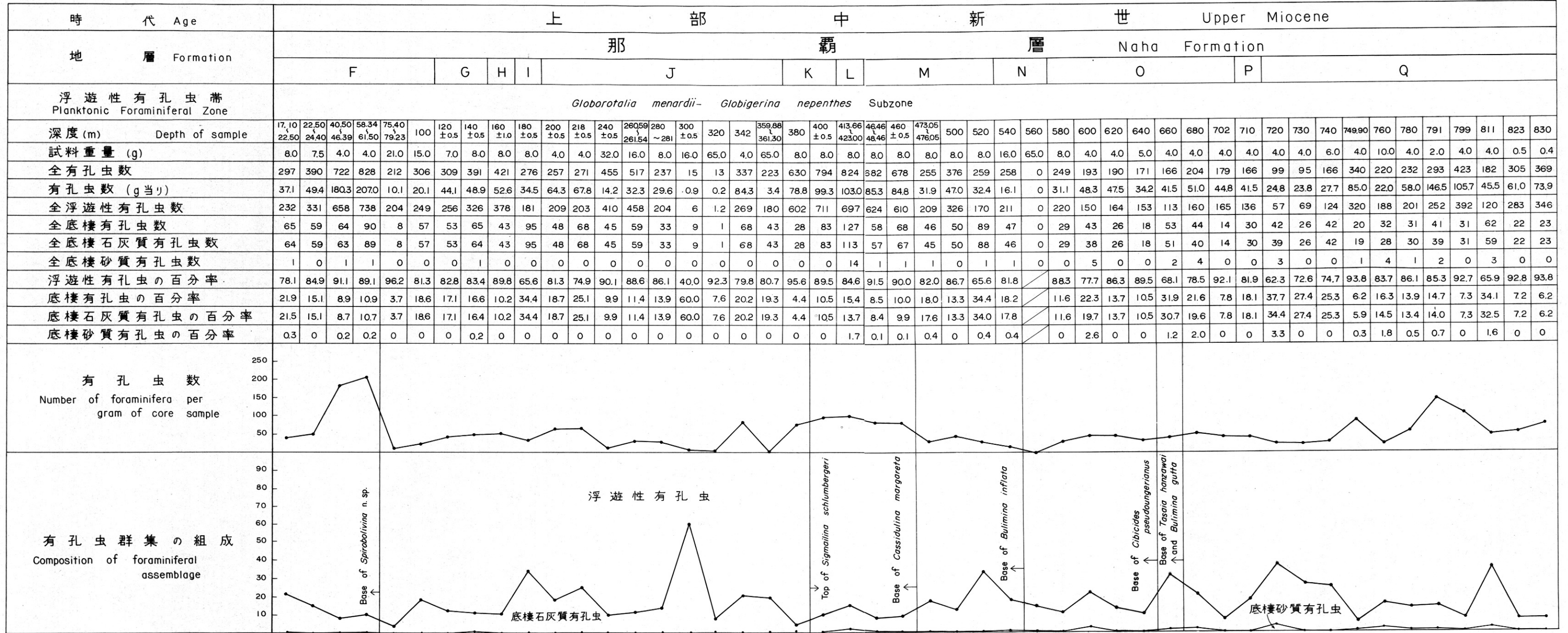
第15表 那覇2号井における島尻層群下部の有孔虫統計表 Statistical table of Foraminifera from the lower part of Shimajiri Group at Naha R-2 Test Well
