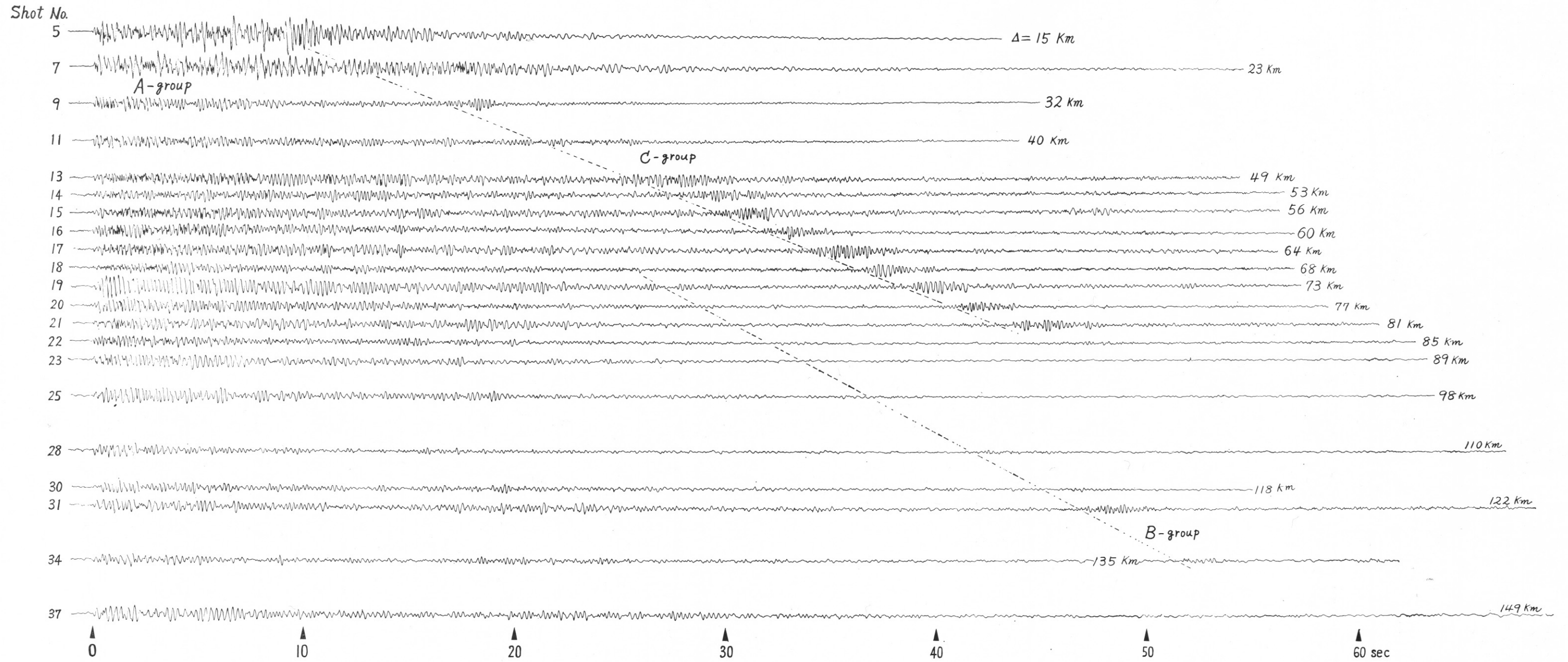
第2図 観測された記録 Seismograms.
