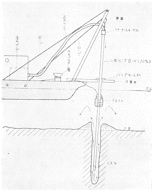
第17図 海底沈積物層厚調査装置
