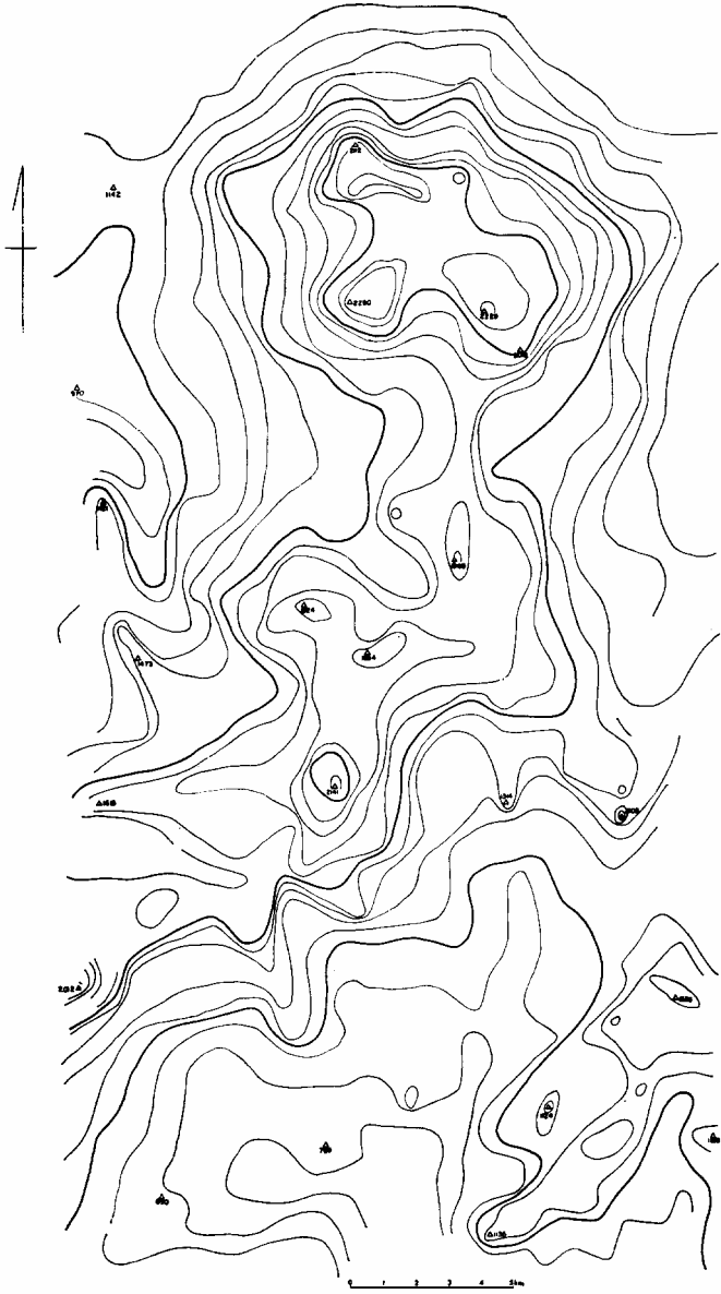
第2图 切 峰 面 图
