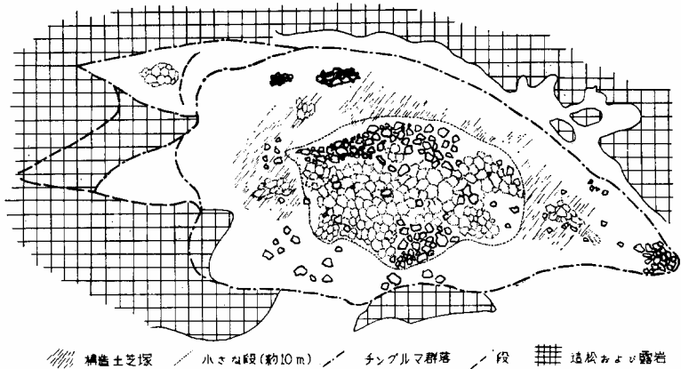
第11図 トムラウシの多角形土
