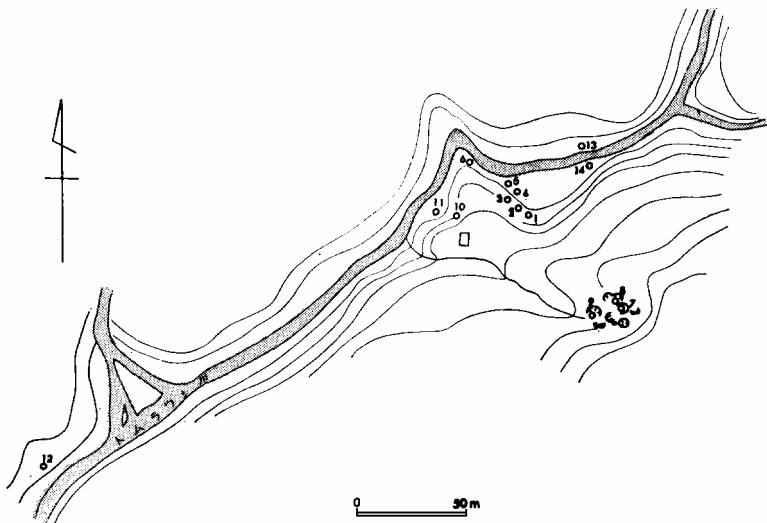
第21図 トムラウシ地獄付近の温泉分布図
