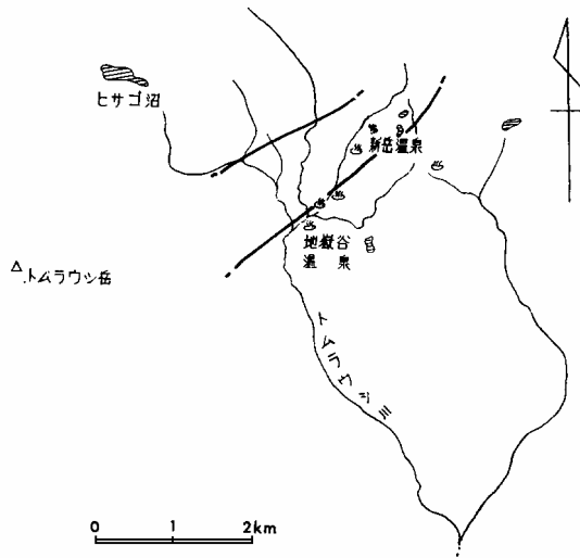
第20図 トムラウシ地区の温泉分布図
