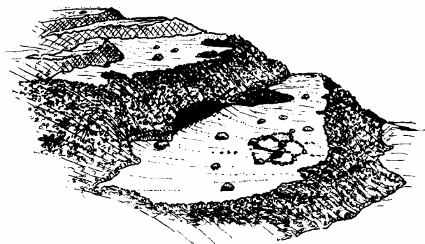
第17図 流土階段
