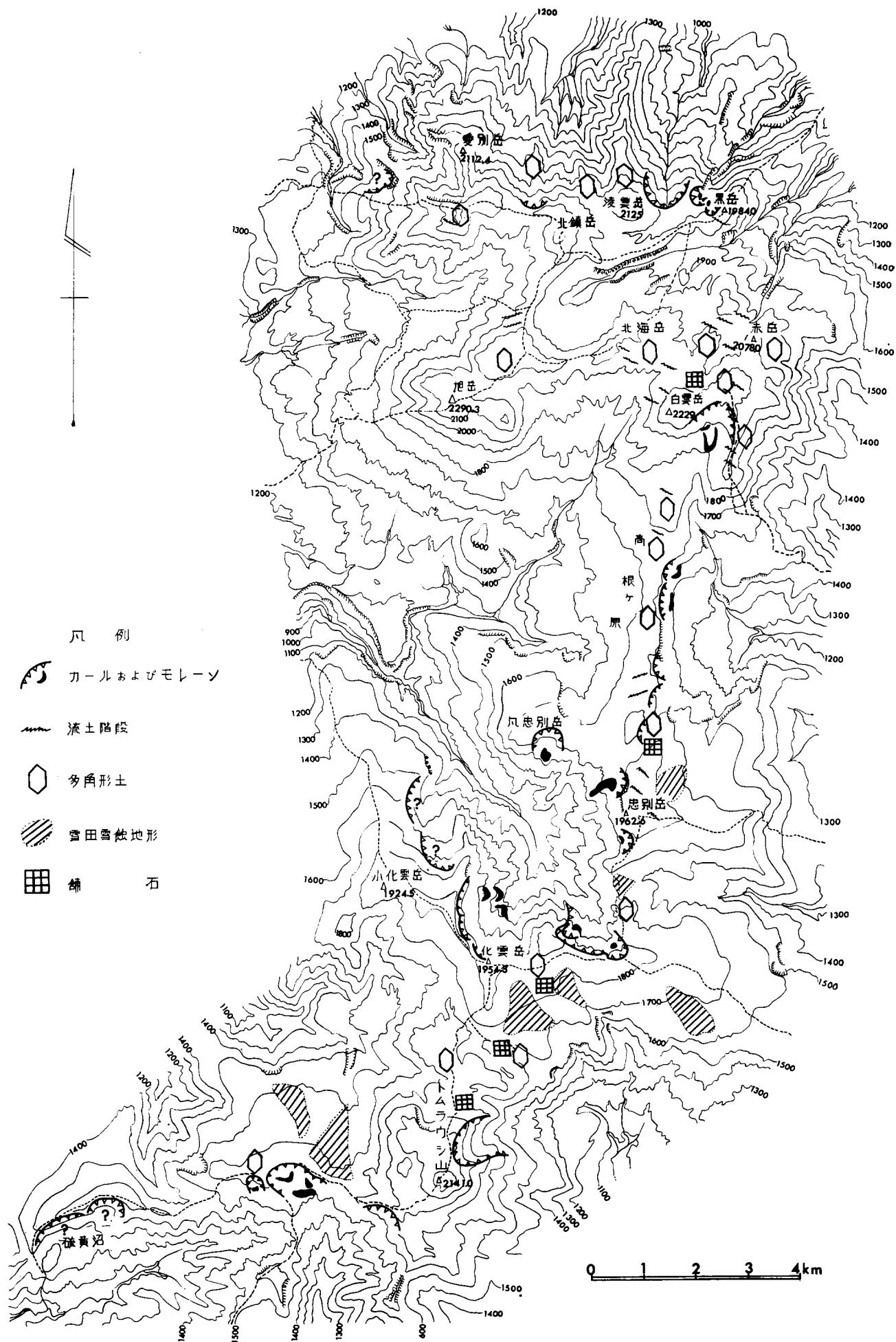
第6図 氷蝕地形および周氷河地形分布図
