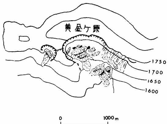
第7図 黄金ヶ原カール
