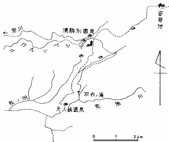
第18図 天人峡および湧駒別温泉分布図
